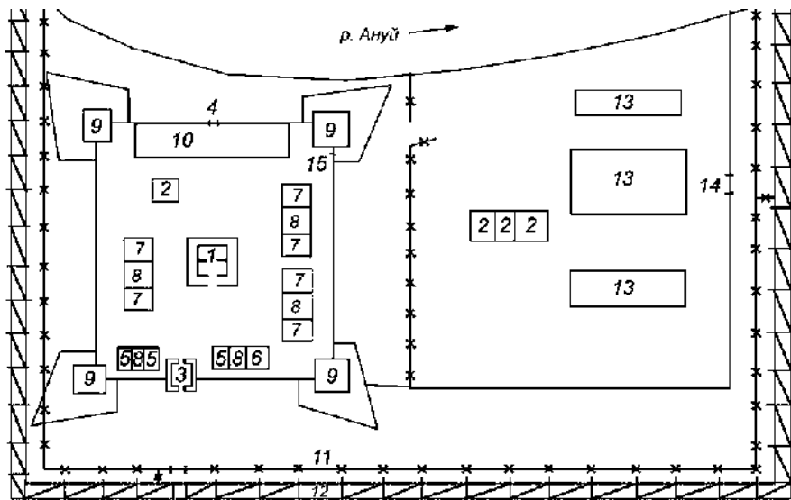
Рис. 4. Схема Ануйской крепости, проект модернизации 1756 г. 1 – пороховой погреб; 2 – провиантский амбар; 3 – ворота, над ними башня; 4 – малые ворота; 5 – офицерские светлицы; 6 – при них черные избы; 7 – казармы; 8 – бани; 9 – надлежит переправить бастионы; 10 – конюшня; 11 – рогатки; 12 – надолбы; 13 – собственные драгун и казаков дома; 14 – заплот; 15 – потайная калитка из крепости.
