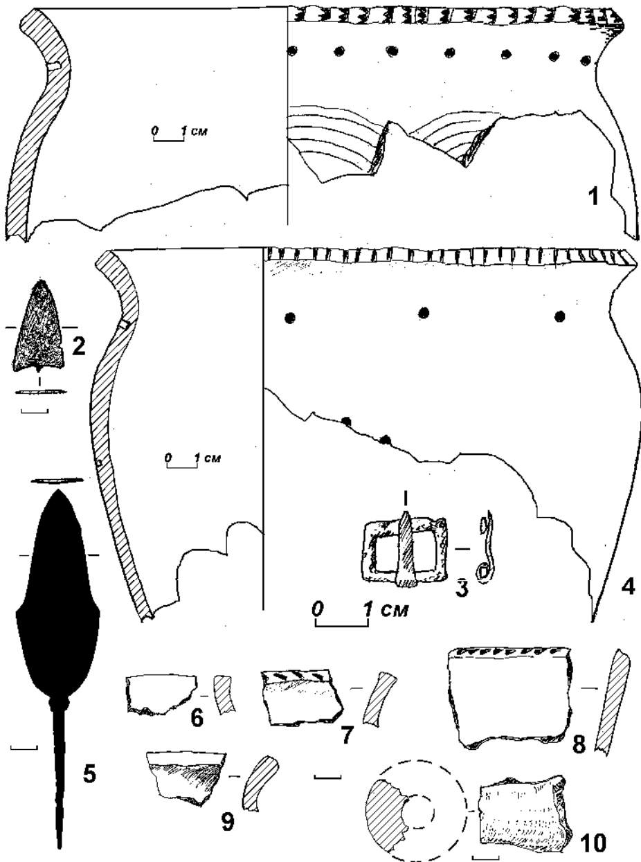
Рис. 14. Усть-Пызас 2. 2, 5 — железо; 3 — бронза, железо; остальное — глина.
