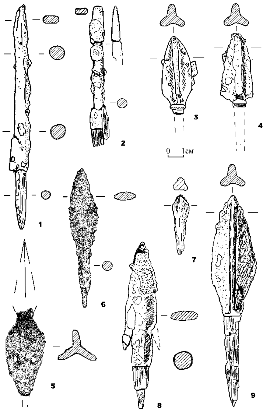
Рис. 1. Шестаки-II. 1-9 — наконечники стрел. Всё — железо.
