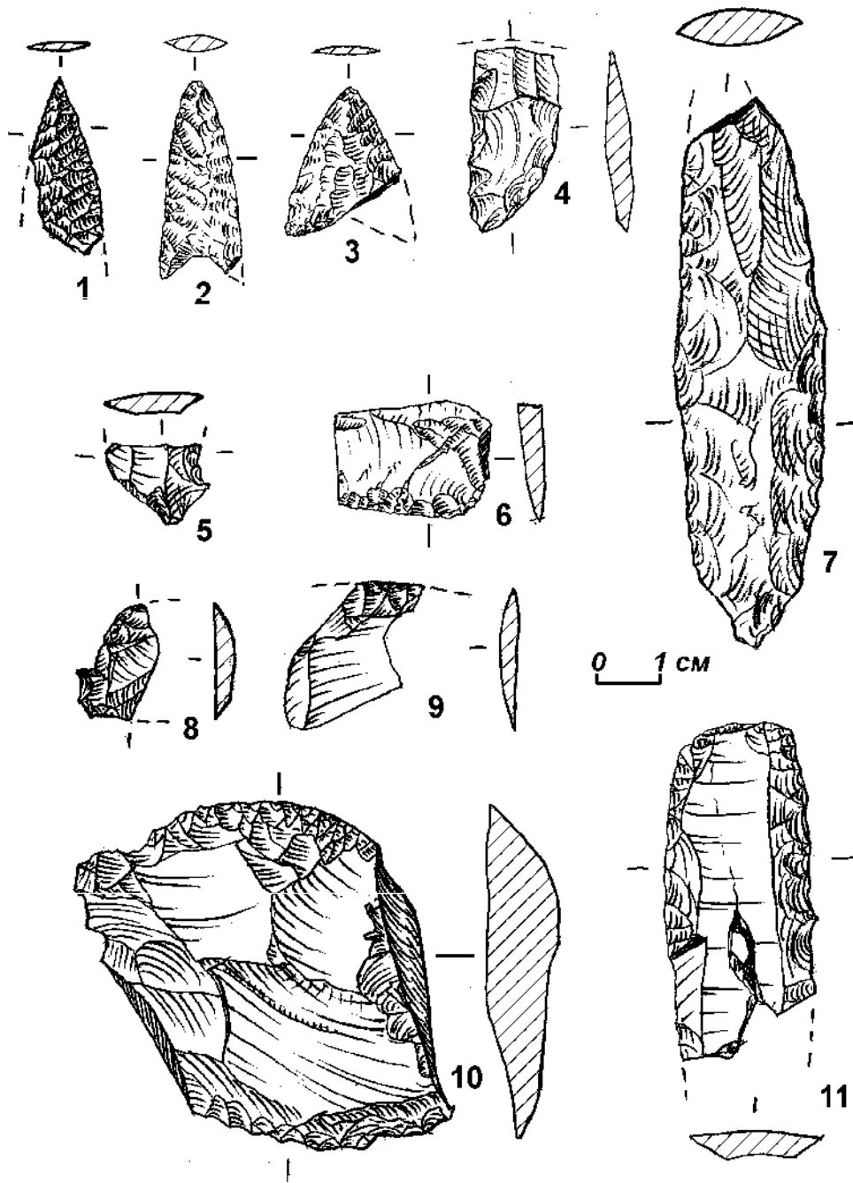
Рис. 8. Усть-Пызас 2. Всё — камень.
