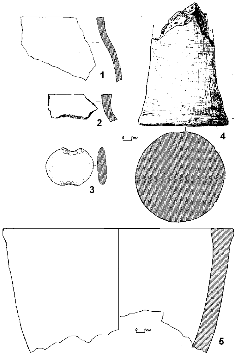
Рис. 7. 1-4 — поселение Казас; 5 — поселение Камешок. 3 — камень, остальное — глина.
