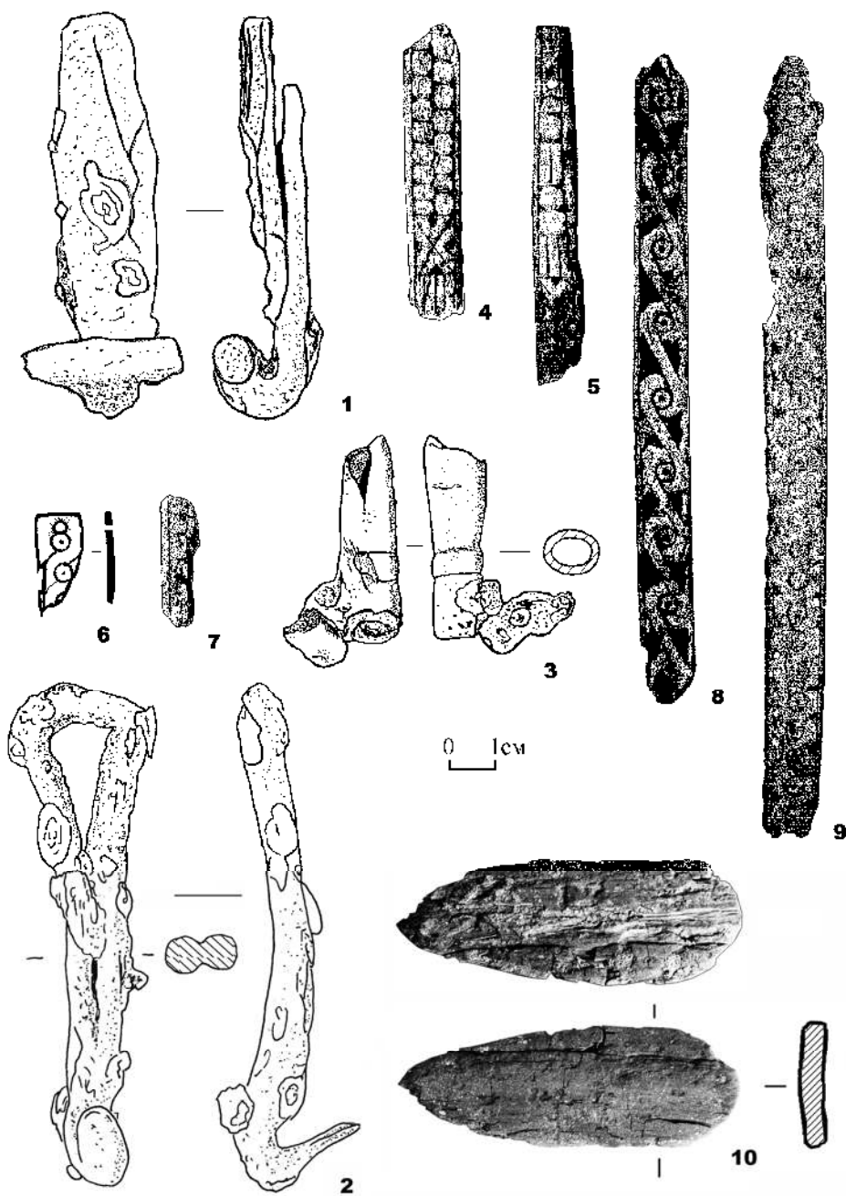
Рис. 6. Шестаки-II. 1-2 — колчанные крюки; 3 — игольник в форме колчана для стрел (расплавлен); 4-9 — декоративные накладки колчана; 10 — донце колчана. 1-2 — железо; 3 — бронза; 4-8 — кость; 10 — дерево.
