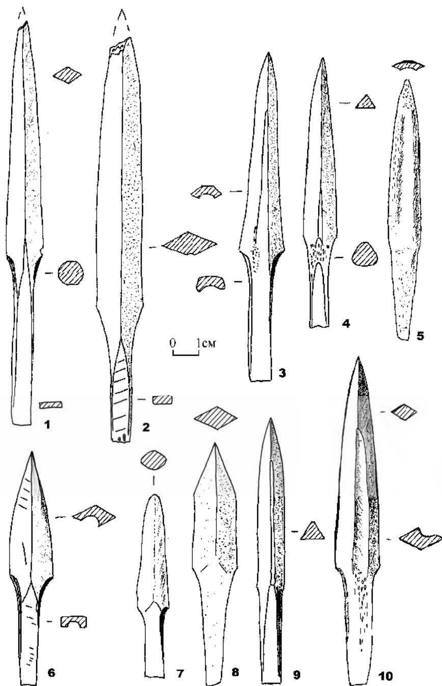
Рис. 3. Шестаки-II. 1-10 — костяные наконечники стрел.
