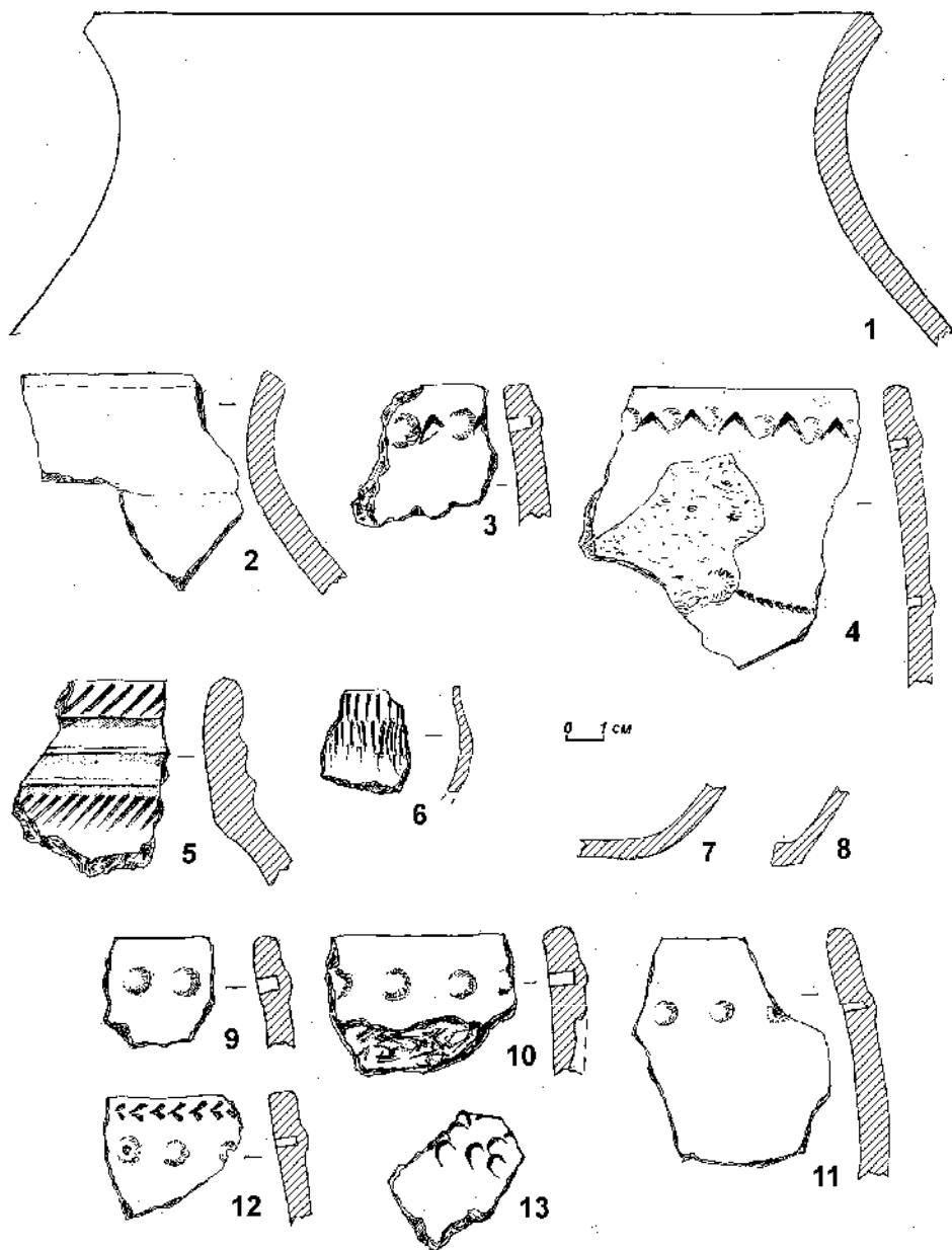
Рис. 11. Усть-Пызас 2. Всё — глина.
