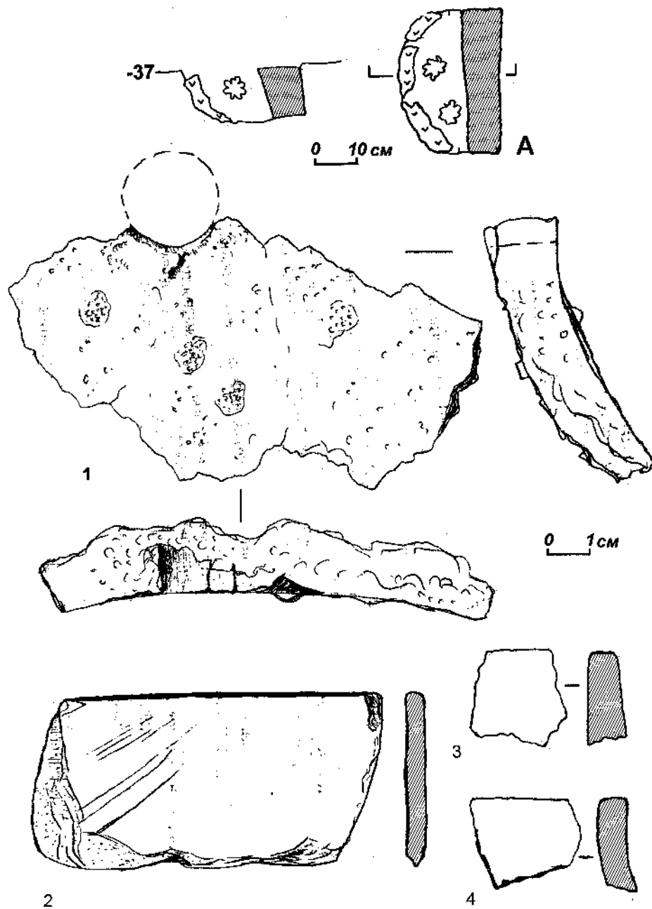
Рис. 6. Поселение Першин Лог. А — разрез и план остатков железоплавильной печи; 2 — камень, остальное — глина.
